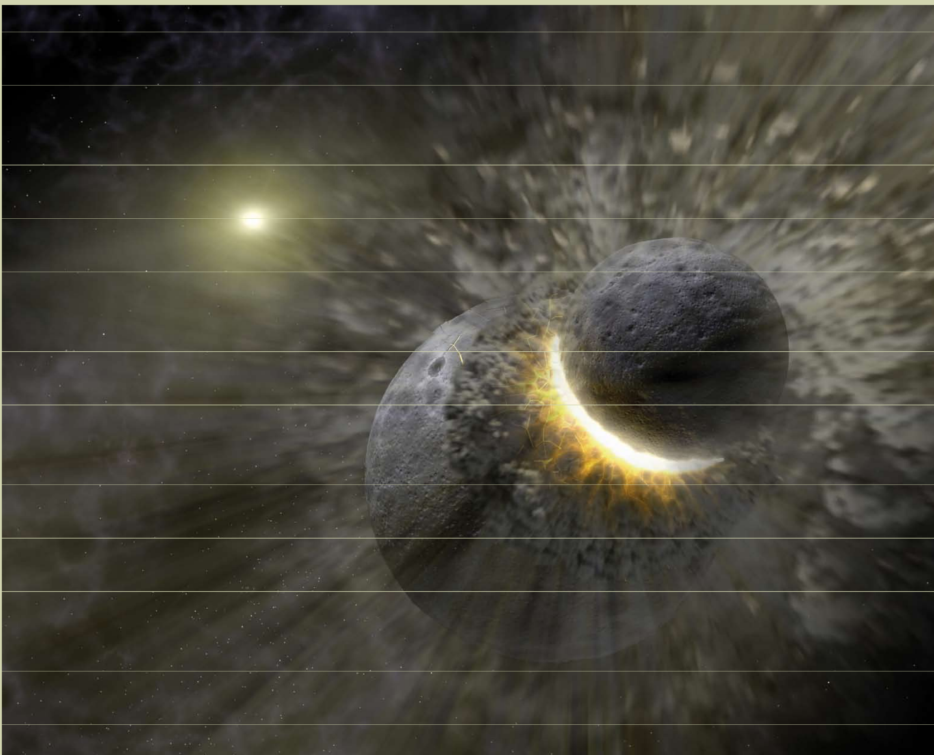
Billard cosmique: la formation de la Terre et de la Lune. Pendant plusieurs dizaines de millions d'années après sa naissance, de nombreuses collisions, notamment entre objets de masse planétaire, ont agité le système solaire. Certains débris ont pu rester au moins partiellement en orbite autour de l'un des objets et se rassembler à nouveau pour former un nouveau corps satellite du premier: c'est ainsi que l'on comprend aujourd'hui la naissance de la Lune, environ 70 millions d'années après le début de la formation du système solaire. [Dessin d'artiste © NASA]
