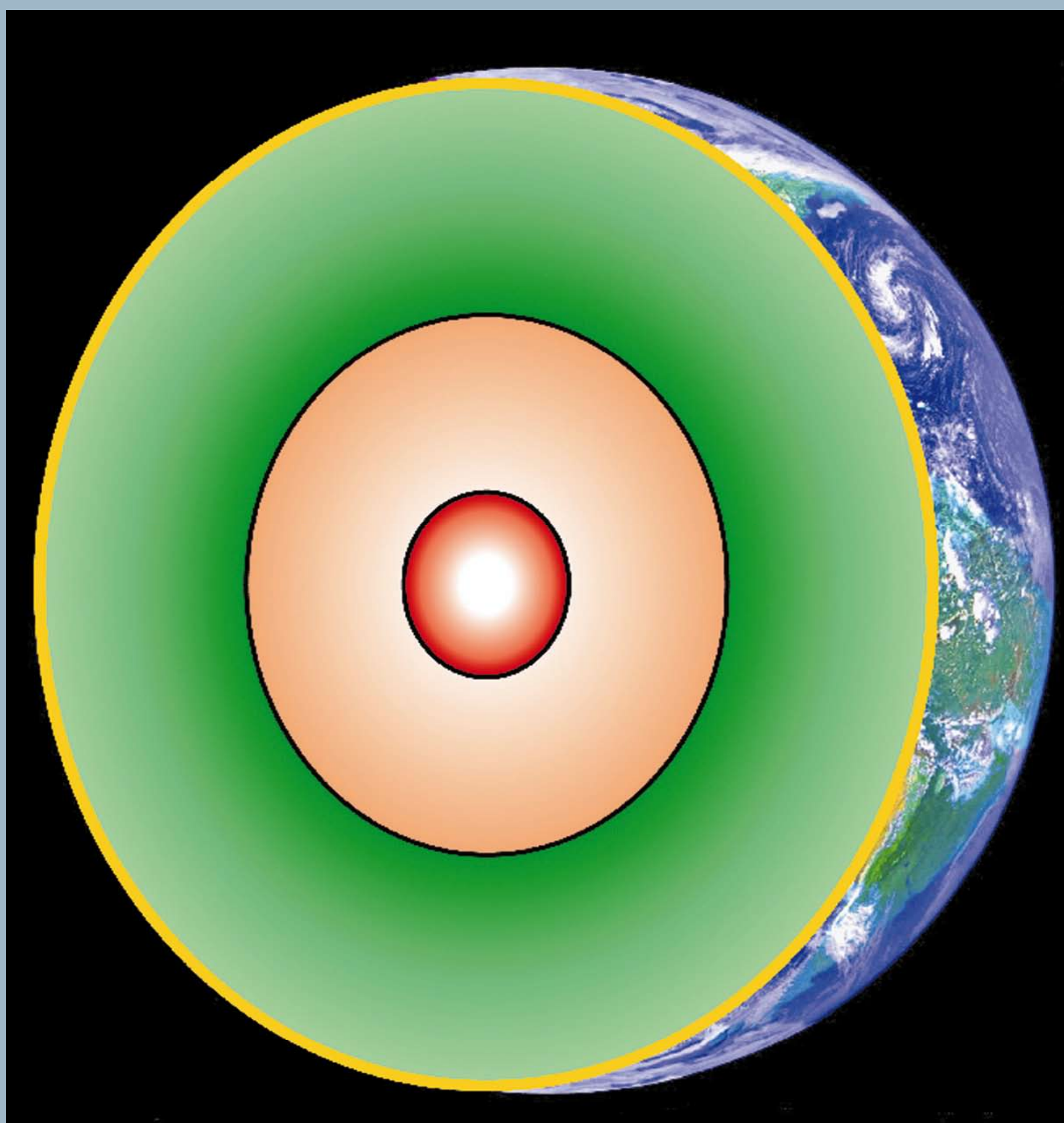
Coupe schématique de la Terre solide actuelle montrant sa structure en couches concentriques : rouge foncé = noyau interne solide; rose orange = noyau externe liquide; vert = manteau; jaune = croûtes océanique et continentale.
