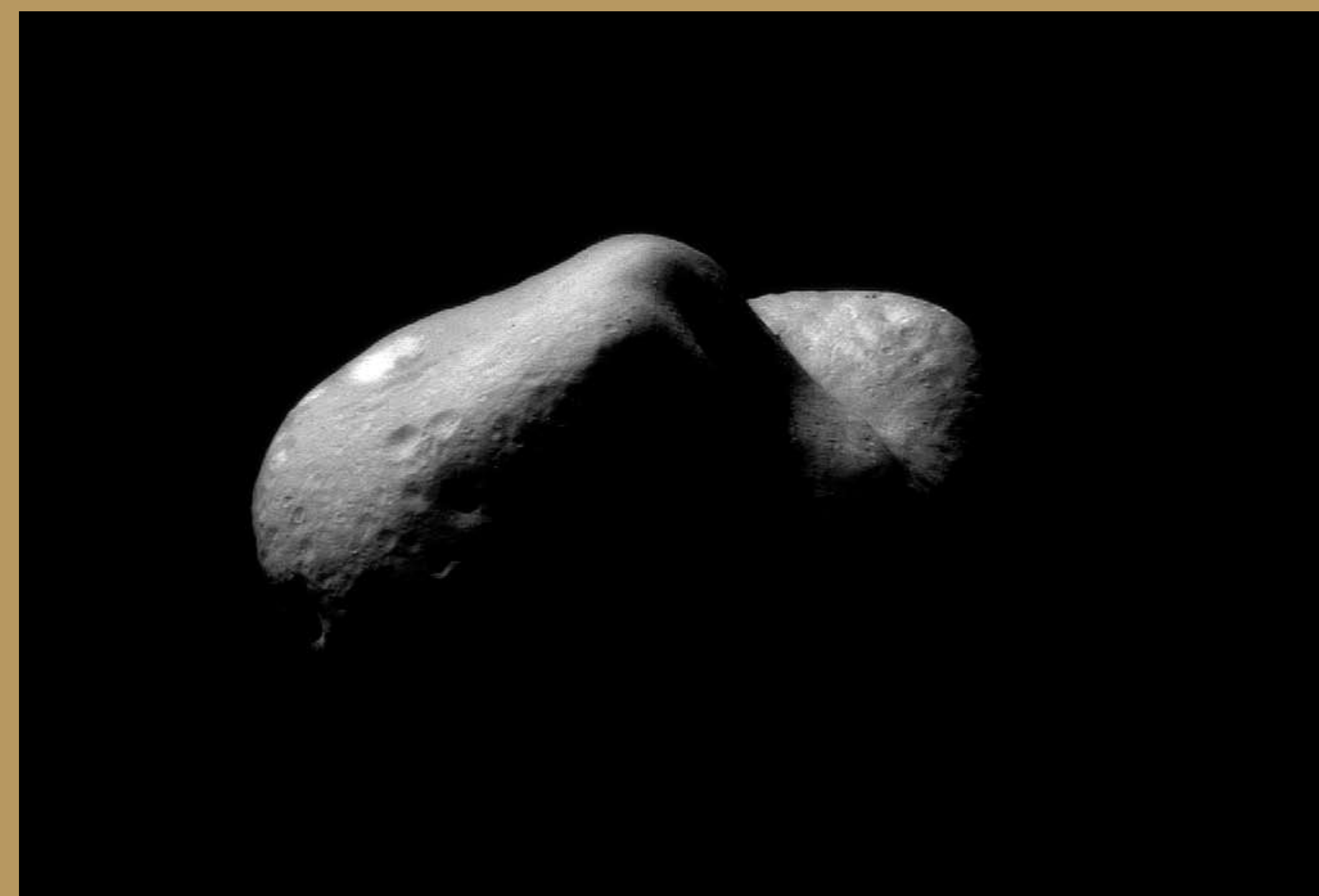
L'astéroïde appelé 433 Eros a été survolé le 19 septembre 2000 par la sonde américaine "NEAR-Shoemaker". Ce "petit corps" du système solaire (33 km de long) fait aujourd'hui partie de la "ceinture d'astéroïdes", qui en comprend des millions. De tels astéroïdes, alors situés suffisamment loin du Soleil pour contenir beaucoup de glace, ont probablement participé à la formation de la Terre, lui apportant jusqu'à un tiers de son eau, suivant de récentes estimations. D'autres corps comme les comètes ou les météorites ont pu également contribuer à l'apport d'eau sur la Terre, mais de façon minoritaire.
