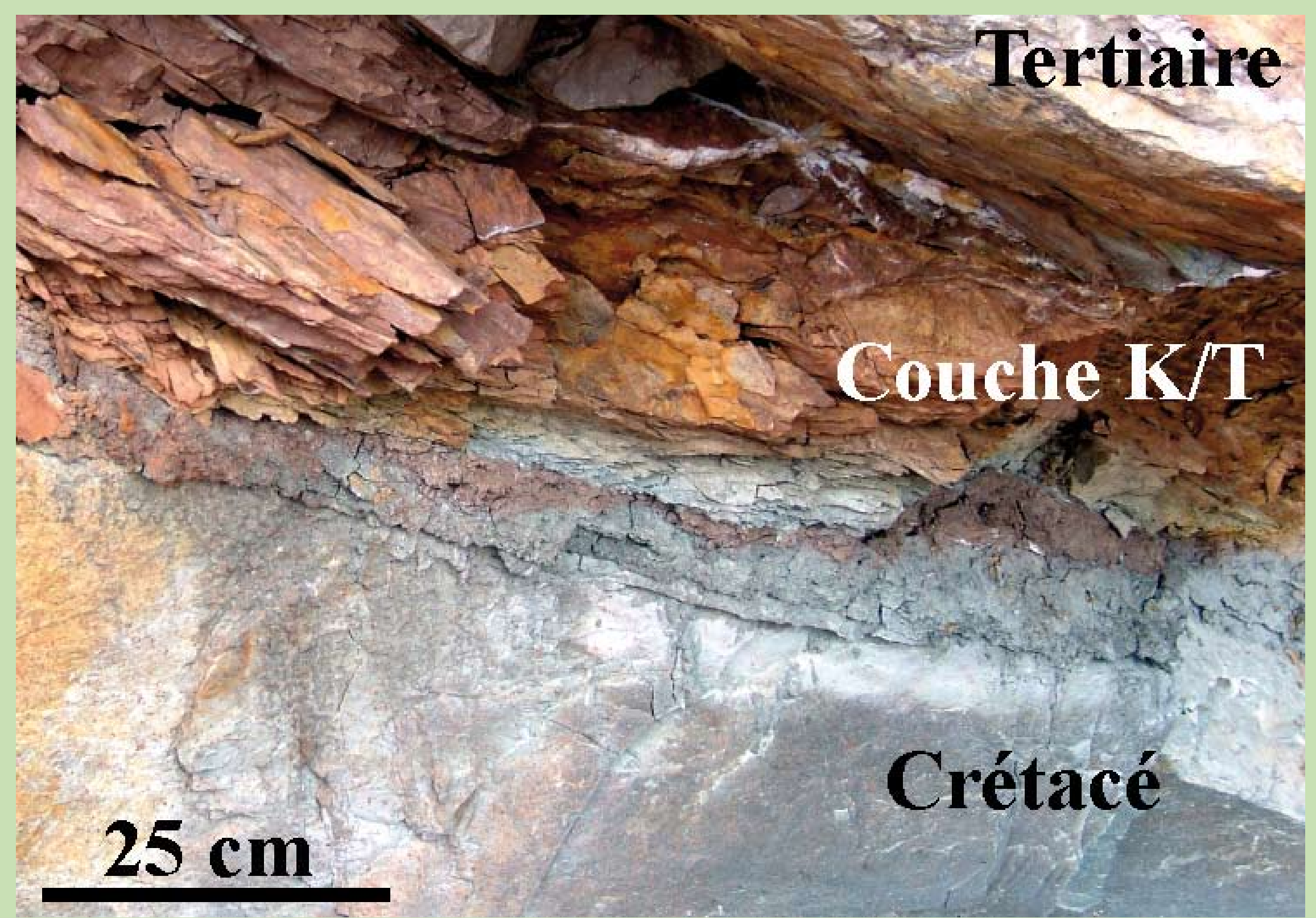
Photo de la limite Crétacé - Tertiaire (couche KT) dans les falaises de la baie de Loya à Hendaye. Contrairement aux deux couches qui l'entourent, cette couche feuilletée de 10 cm d'épaisseur de couleur rouge ocre, est extrêmement riche en iridium. Cet élément de la famille du platine est d'origine extraterrestre. Il a été apporté par la chute de la météorite de Chicxulub dans la presqu'île du Yucatan. Cet impact a provoqué un cataclysme planétaire à l'origine des grandes extinctions (dinosaures, ammonites, etc) observées au passage Crétacé - Tertiaire.
