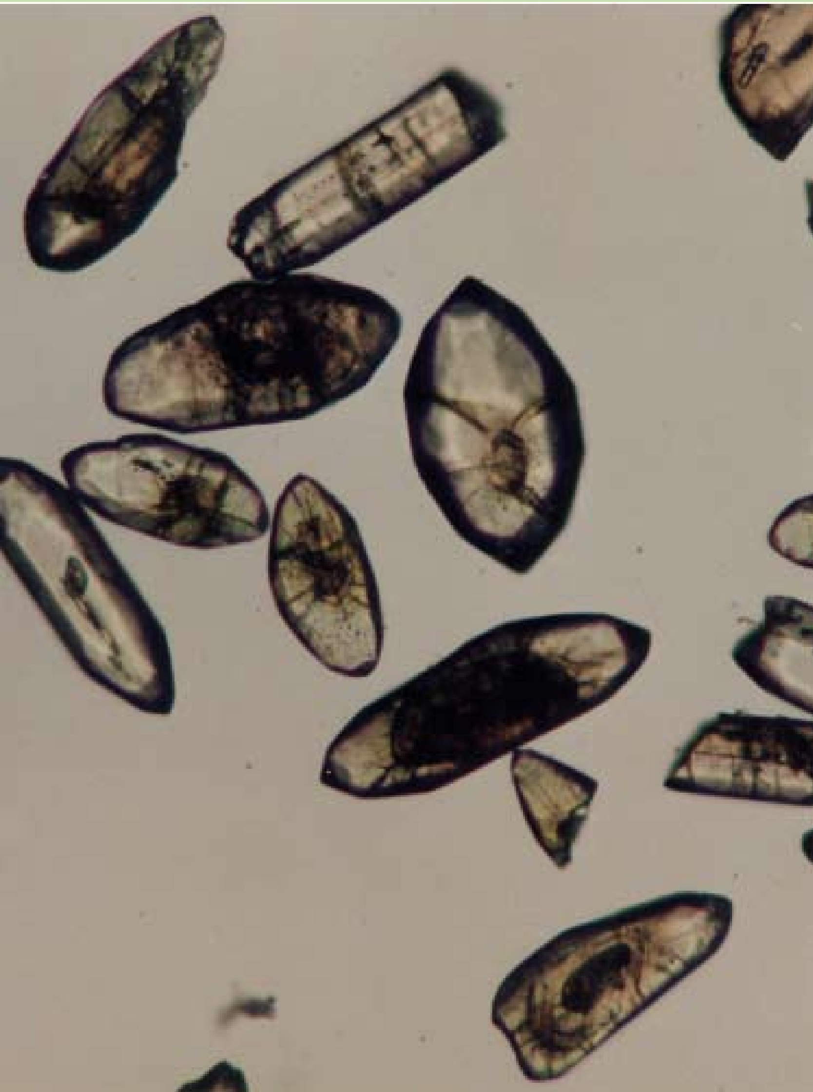
Cristaux de zircon archéens semblables aux cristaux découverts à Jack Hills en Australie. Ces minéraux de formule (Zr SiO 4 ) qui se forment de préférence dans des magmas granitiques, sont très résistants à l'altération et contiennent aussi des éléments radioactifs tels que le thorium et l'uranium, qui permettent de les dater aisément. Ce sont d'excellents mémoires de l'histoire terrestre.
